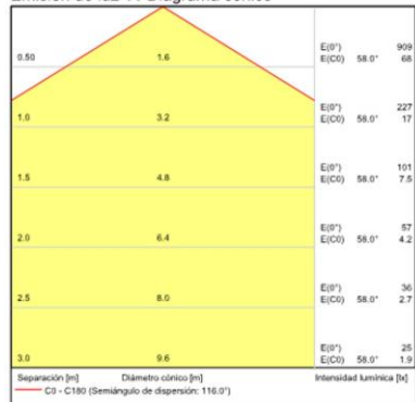
Emisión de luz 1 / Diagrama conico
