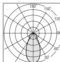
Diagramma Polare (50°)
