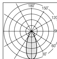
Diagramma Polare (30°)
