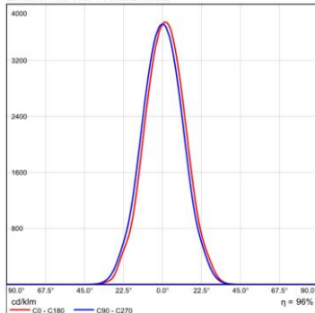
Emisión de luz 1 / CDL lineal
