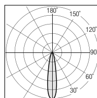
Diagramma Polare (16°)
